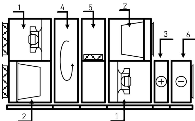
Рисунок 2 - Функциональная схема VERSO R
