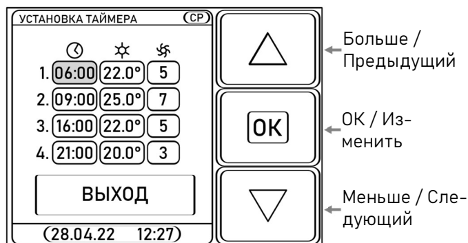
Рисунок 11 - Экран подменю установки таймеров
