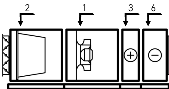
Рисунок 1 - Функциональная схема VERSO S
